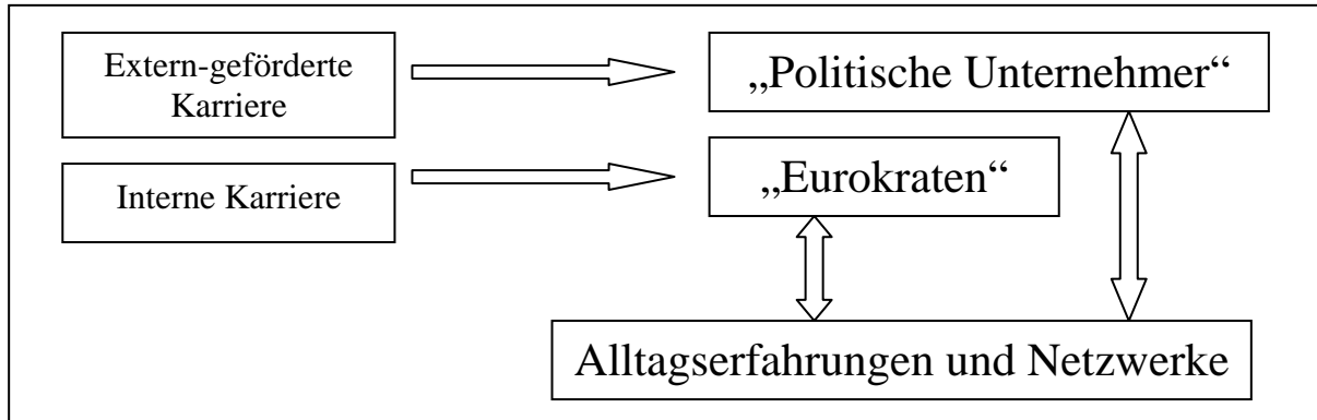
Abb. 3: Spaltungsthese
