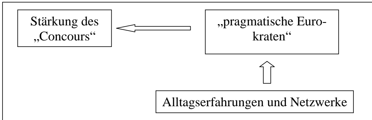
Abb. 4: Homogenisierungsthese
